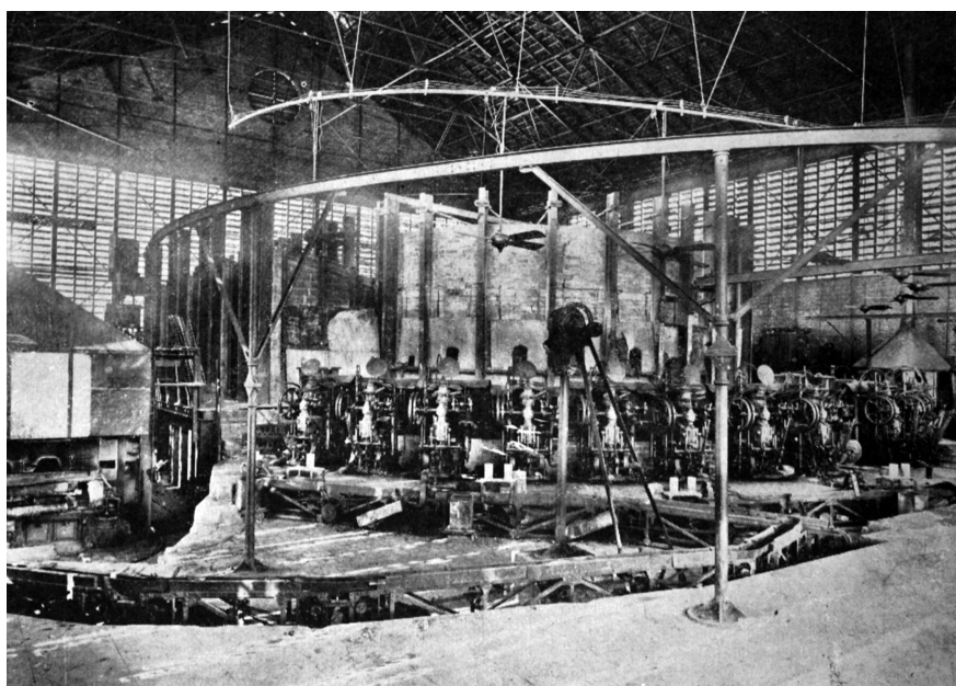
FIGS. 6-9. Vidraria Santa Marina. Vistas da fachada e dos fundos da fábrica e vistas externa e interna dos fornos de garrafa, [1916].
